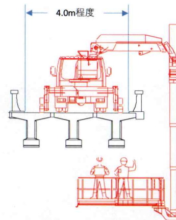
橋梁点検車 正面(イメージ図)
