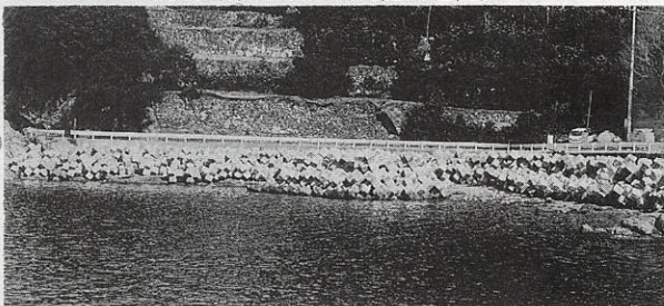
高潮対策として(大佐田地区)
