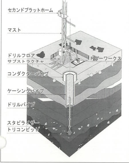
温泉掘削装置の稼働状況図
