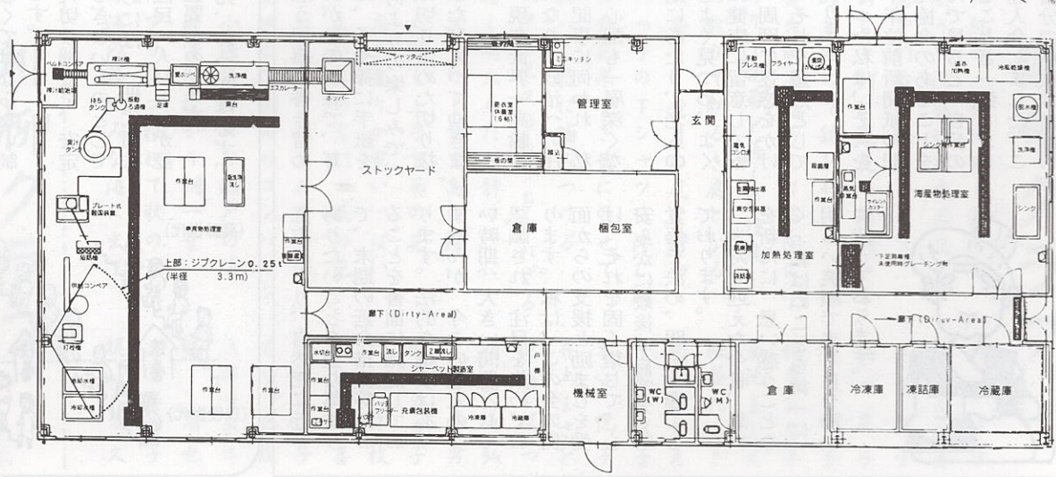
〔農水産物処理加工施設平面図〕
