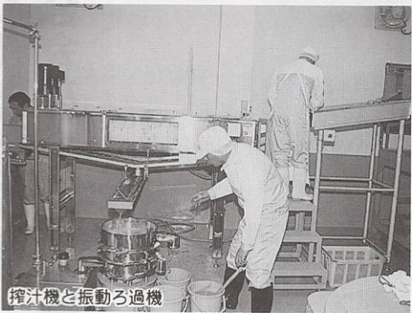
搾汁機と振動ろ過機
