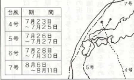
今年発生した台風の進路図
