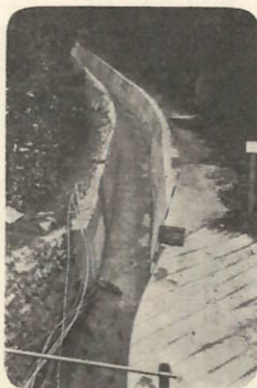
(4) 湊浦寺川排水路整備 延長129.5m 幅員10.7m~4m 事業費 4,460千円 (交付金4,400千円)
