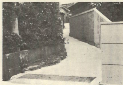
(7) 川永田神社線舗装(コンクリート舗装) 延長119m 幅員1.5m~2.4m 事業費 790千円(交付金700千円)
