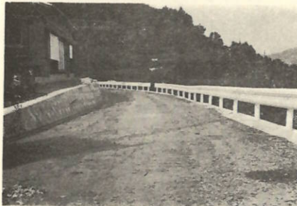
(13) 町道九町二見線新設 延長 124.4m 幅員 4m 事業費 31,636千円 (交付金 31,600千円)
