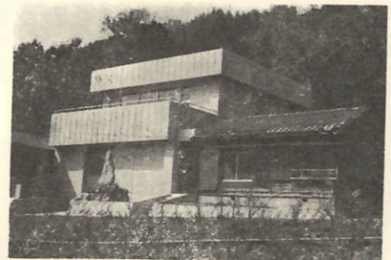
(11) 奥集会所新築 鉄筋コンクリート2階建 198.61㎡ 事業費 13,583千円 (交付金 7,900千円)
