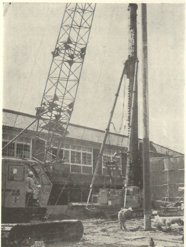
長さ32メートルのコンクリートパイル70本を打ち込む基礎工事が、現在進められています。
