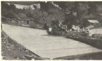
(9) 伊方越漁港船揚場新設 延長18m 幅員27m~29m 事業費 6,450千円 (交付金6,400千円)
