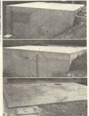
(2)(3)(4) 河内防火水槽 70㎡級 2基 事業費 4,637千円 40㎡級 1基 (交付金 4,600千円)
