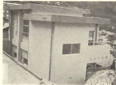
⑪ 亀浦集会所新築 鉄筋コンクリート2階建 延 128.28㎡ 事業費 11,422千円 (交付金 7,400千円)
