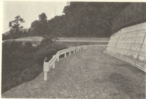
⑬ 町見中央農道新設 延長528m 幅員4m 事業費 55,415千円 (交付金 55,400千円)
