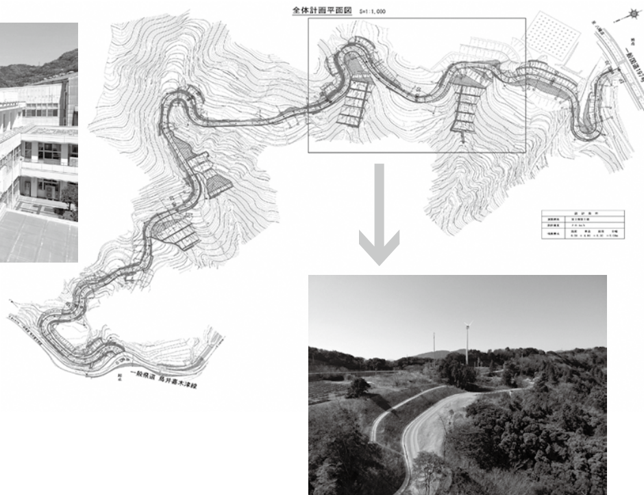
③町道鳥津国道線道路平面図
