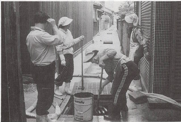
きれいになった下水道(二名津地区)
