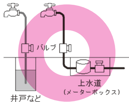
上水道とそれ以外の管がつながれていない。
