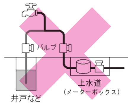
上水道とそれ以外の管が直接つながっている。
