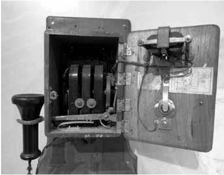
写真3 電話機内部2
